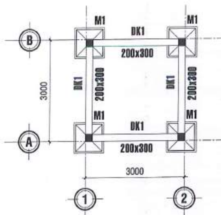
MẶT BẰNG MÓNG, ĐÀ KIẾNG NHÀ RÁC TL 1/100
