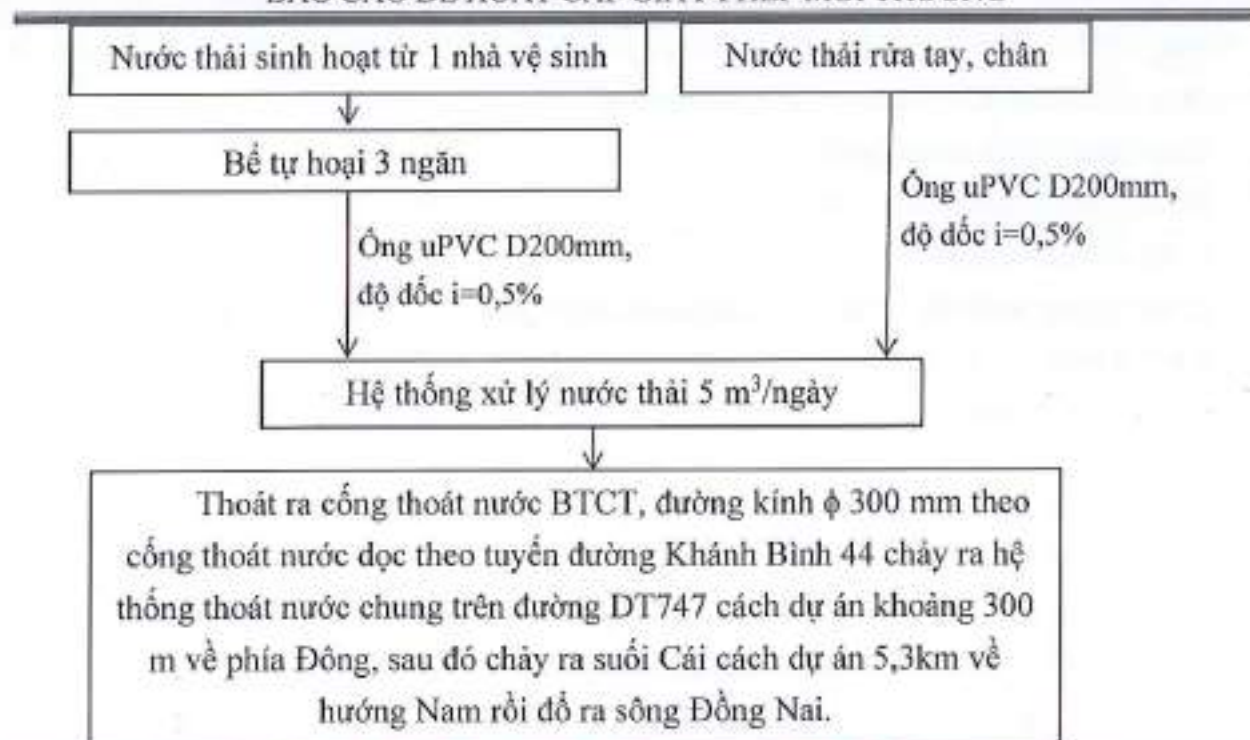
Hình 4.1. Sơ đồ quản lý nước thải của dự án
