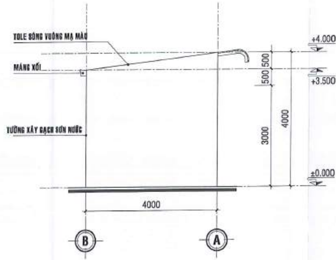
MẶT ĐỨNG TRỰC B - A TL 1/100
