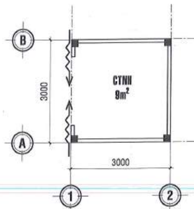
MẶT BẰNG NHÀ RÁC TL 1/100
