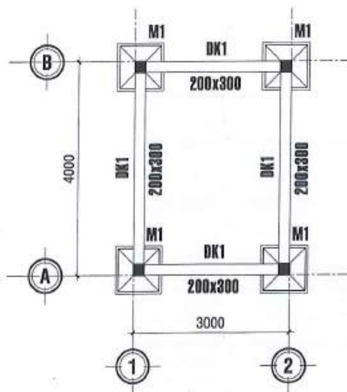
MẶT BẰNG MÓNG, ĐÀ KIỀNG TL 1/100
