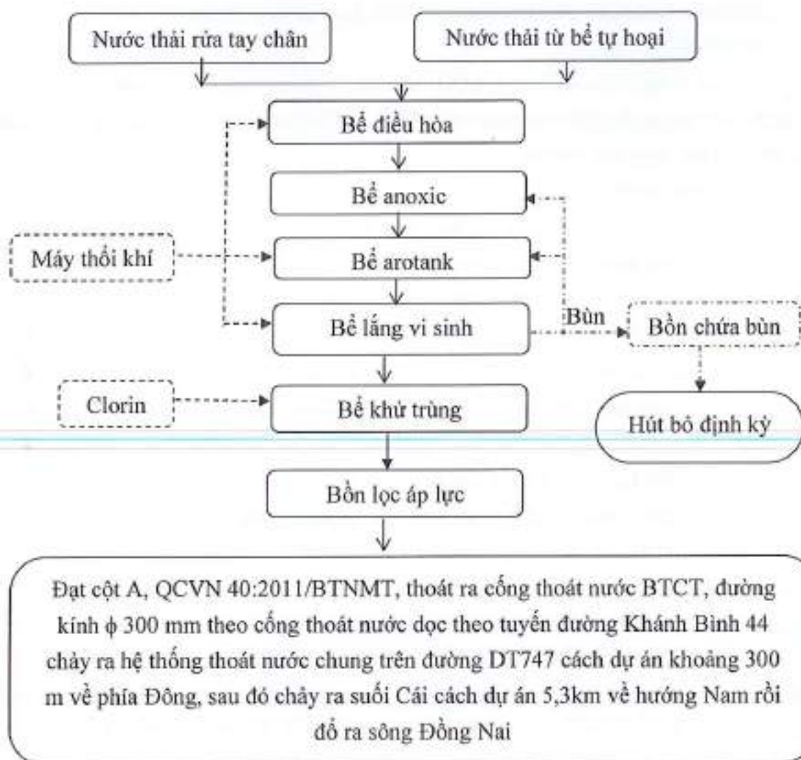
Hình 4.3. Quy trình công nghệ HTXLNT công suất 5 m³/ngày
