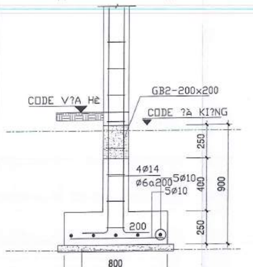
MẶT CẮT 4-4 TL 1/25
