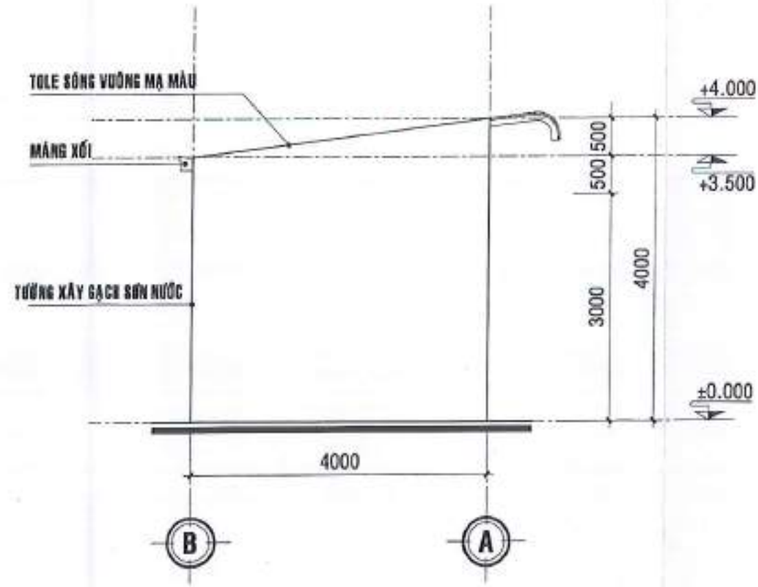
MẶT ĐỨNG TRỤC B - A TL 1/100
